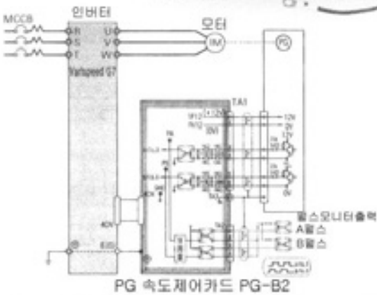
PG 속도제어카드 PG-B2
