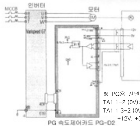
PG 속도제어카드 PG-D2
