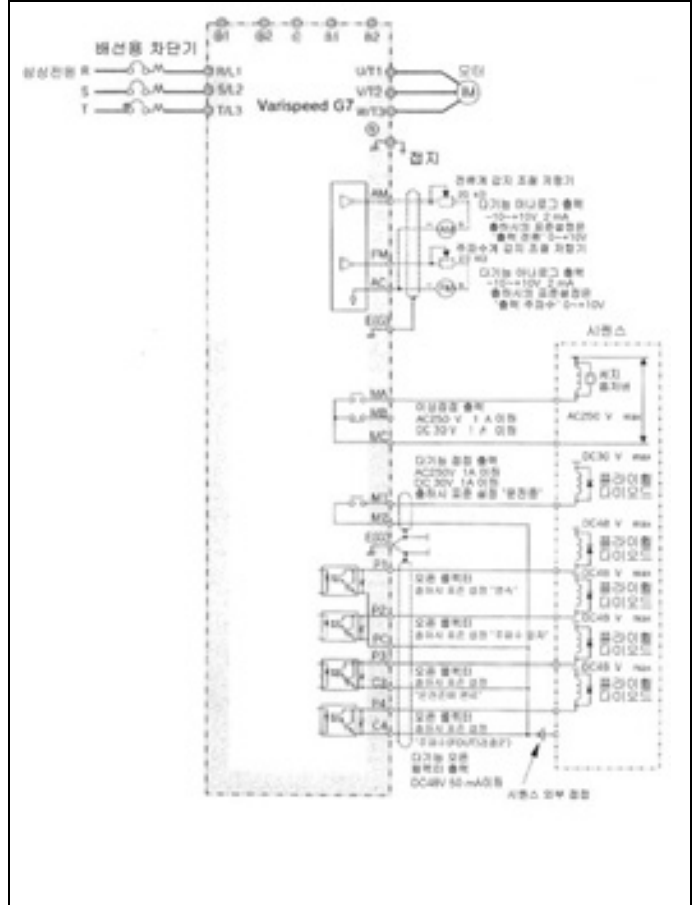
점점 출력, 오픈 컬렉터 출력을 사용할 경우
