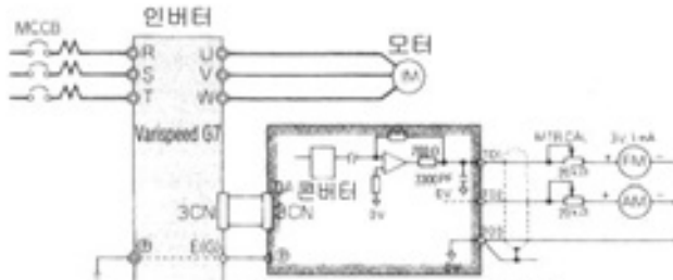
아날로그 모니터 카드 AO-08
