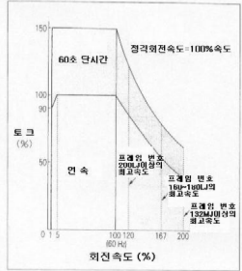
허용부하특성
